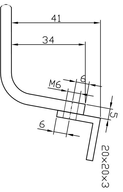
Alternatieve constructie met hoeklijn
